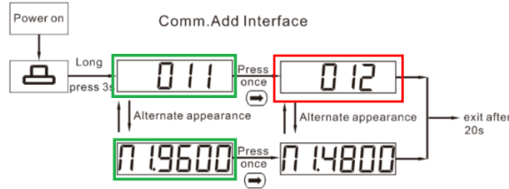
Figura 3.15: procedura di modifica parametri ddsu666-h (meter monofase)
