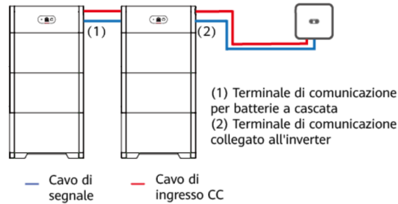
Figura 1.12: connessione dei cavi per il collegamento delle batterie
