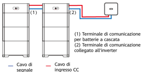
Figura 1.9: connessione dei cavi per il collegamento delle batterie
