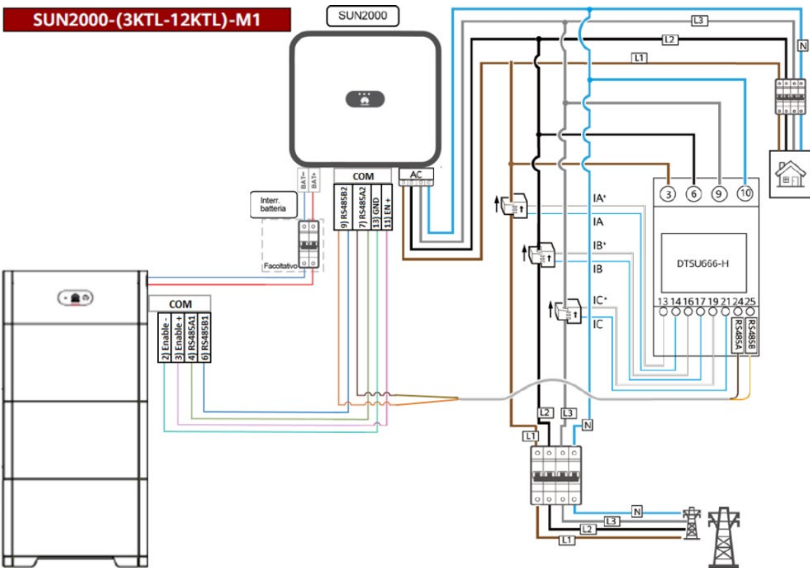
Figura 1.15: schema di connessione dei cavi COM per inverter trifase
