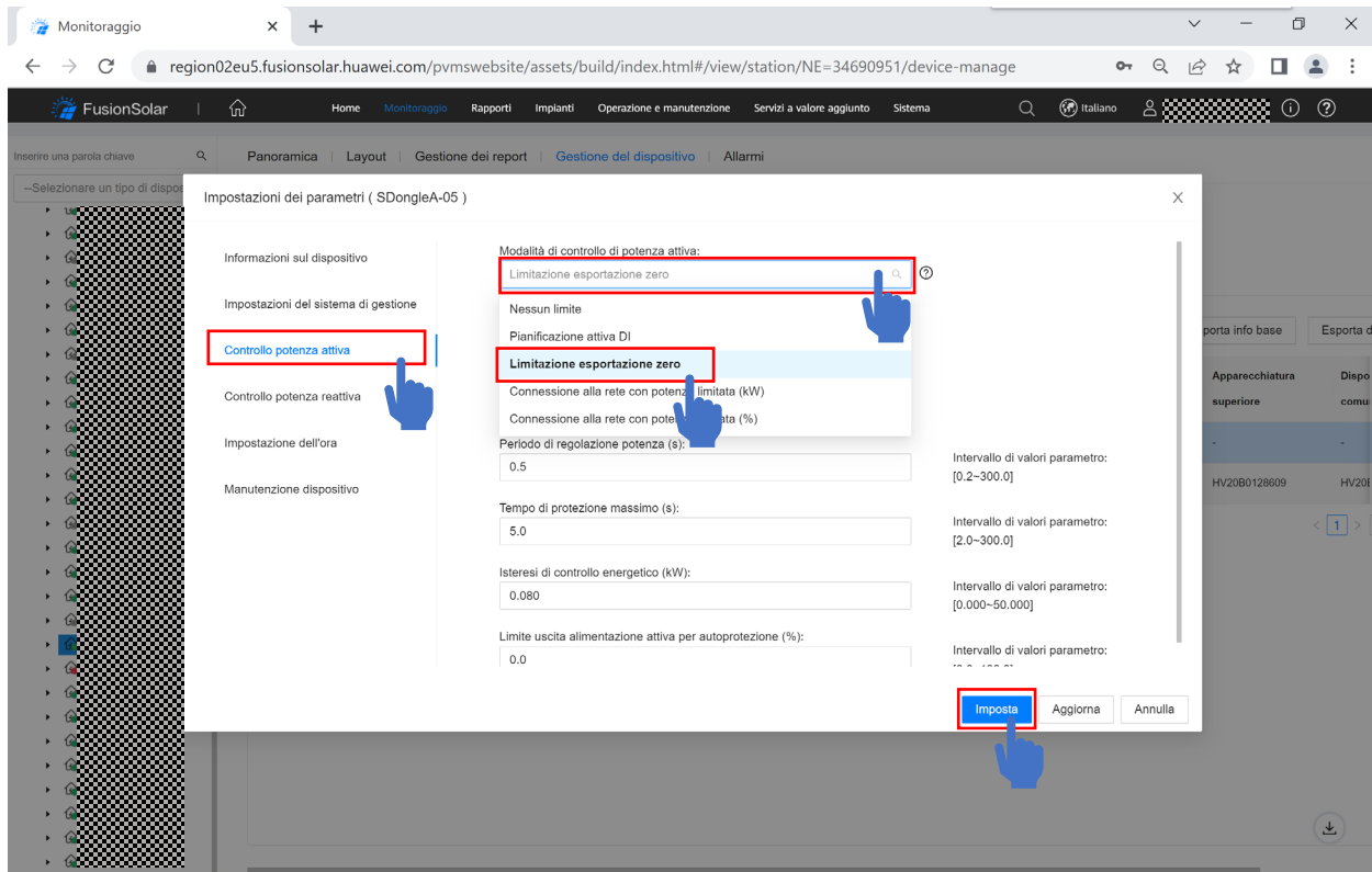
Figura 5.58: immissione zero impianto con Smart Dongle
