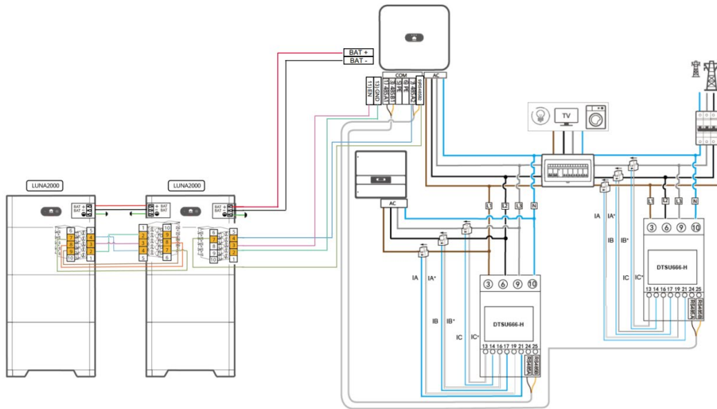
Figura 3.14: schema di collegamento retrofit trifase
