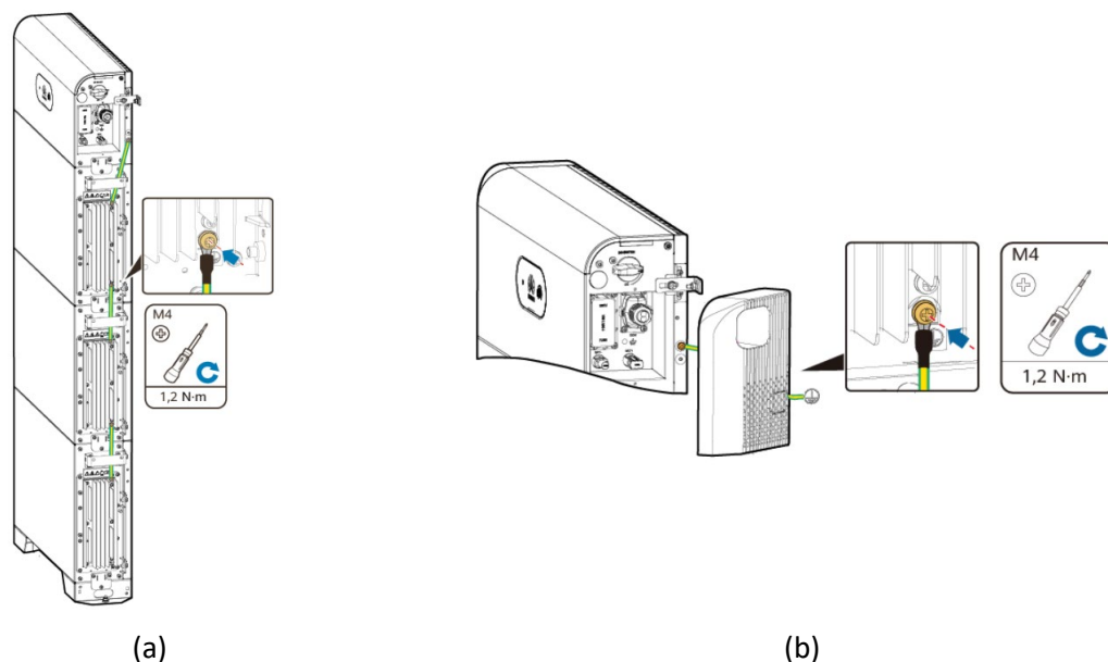
Figura 1.10: messa a terra sulla batteria. (a) moduli di espansione (b) modulo di controllo
