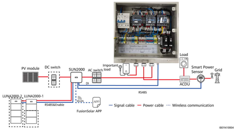
Figura 3.7: collegamento backup-box generico.
