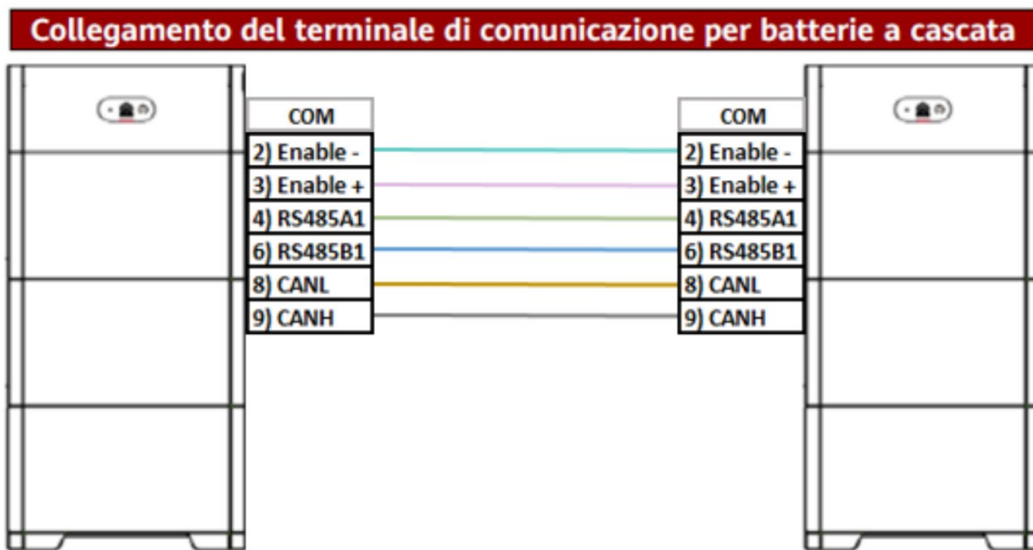
Figura 1.13 schema di connessione dei cavi COM delle batterie
