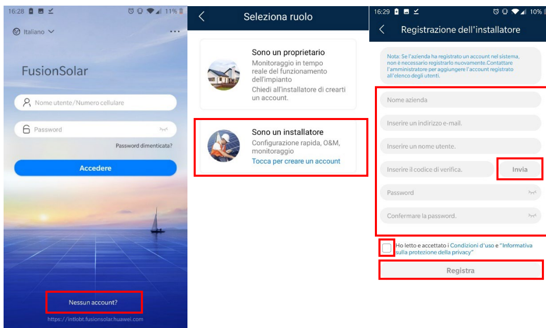
Figura 2.4 Creazione azienda
