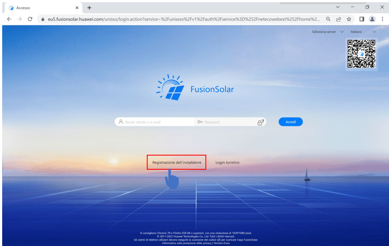
Figura 5.1: registrazione dell'installatore
