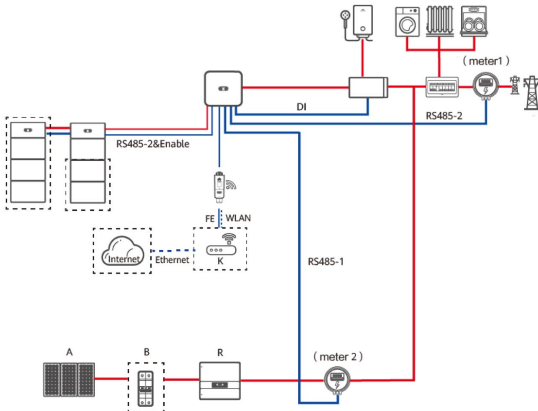
Figura 3.12: schema di configurazione retrofit.
