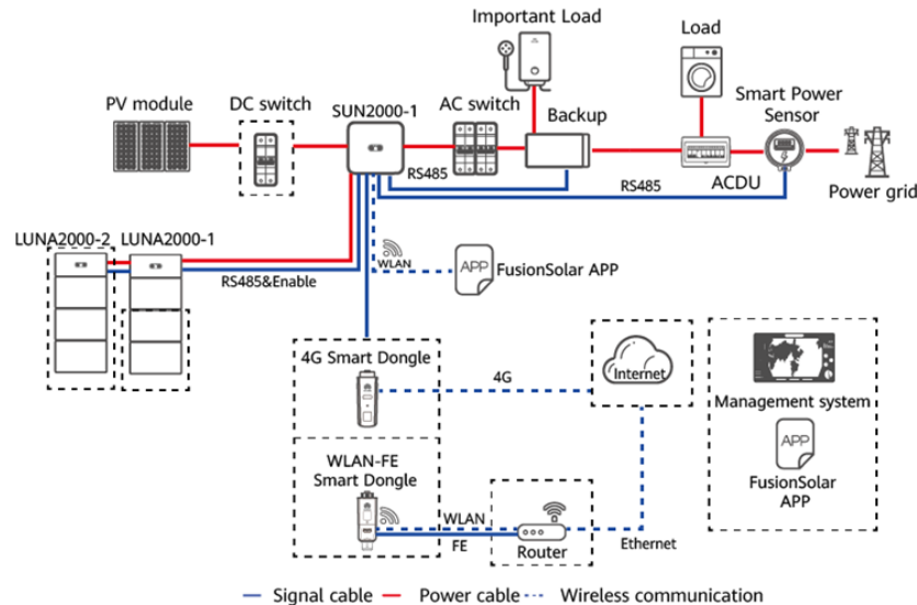
Figura 3.5: configurazione con backup-box
