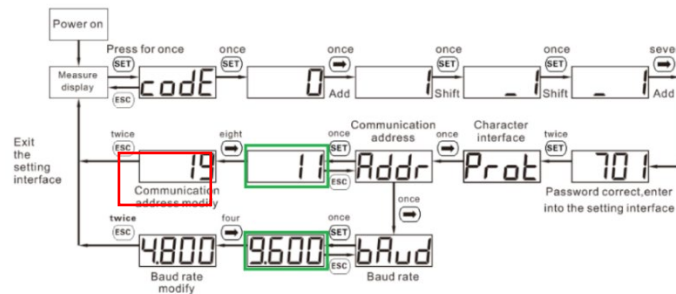
Figura 3.16: procedura di modifica parametri dtsu666-h (meter trifase)
