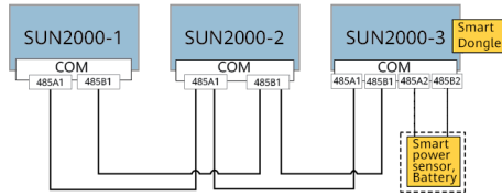
Figura 3.1: schema di collegamento in cascata per inverter monofase
