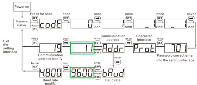
Figura 1.7: procedura di modifica parametri dtsu666-h (meter trifase)
