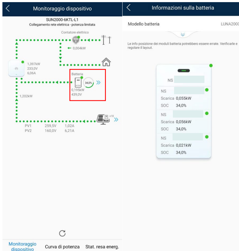
Figura 4.11 Monitoraggio batteria
