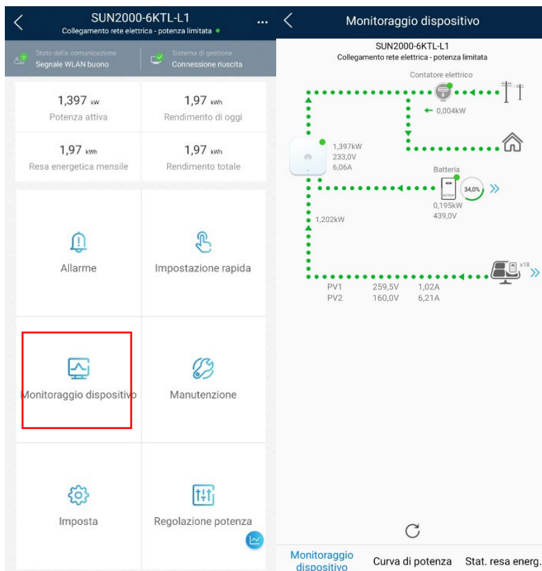
Figura 4.10 Monitoraggio dispositivo
