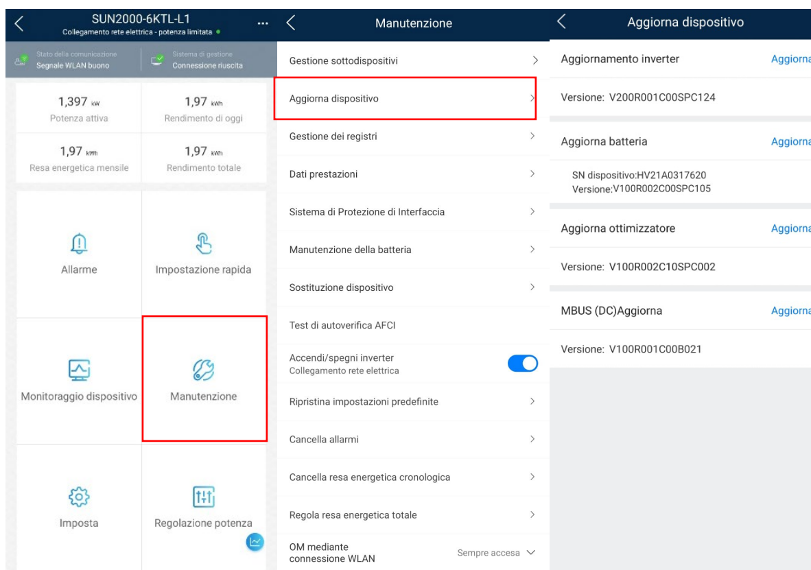
Figura 4.13 aggiornamento dispositivi
