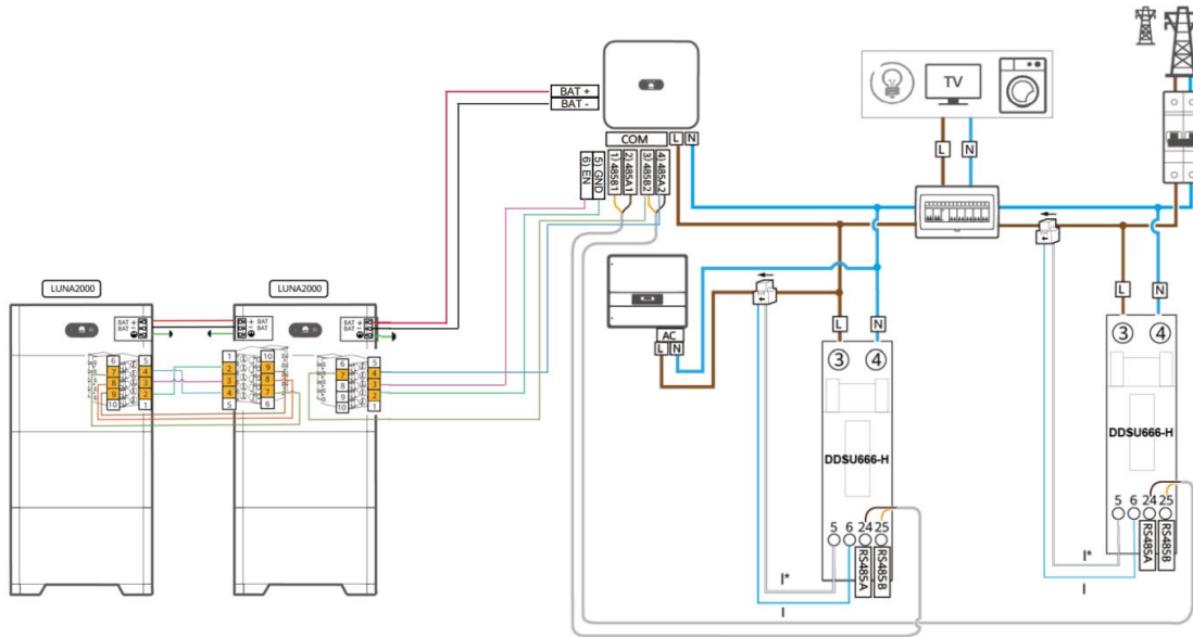
Figura 3.13: schema di collegamento retrofit monofase
