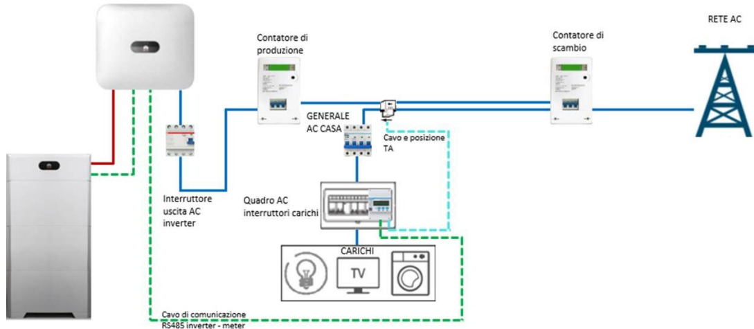
Figura 1.5: schema di posizionamento TA
