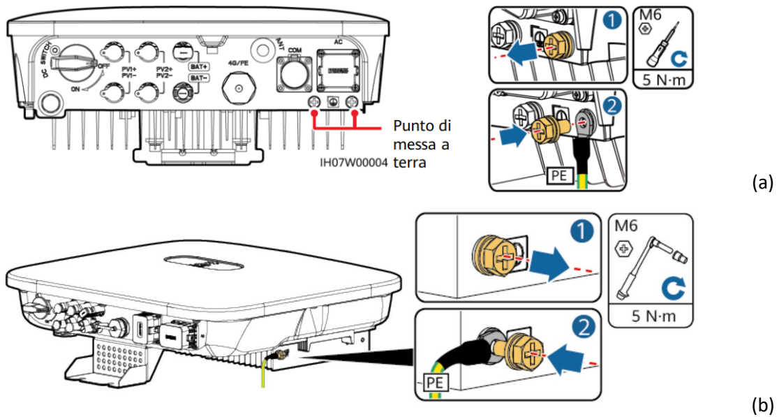
Figura 1.1: punto di messa a terra sulla carcassa. (a) monofase (b) trifase
