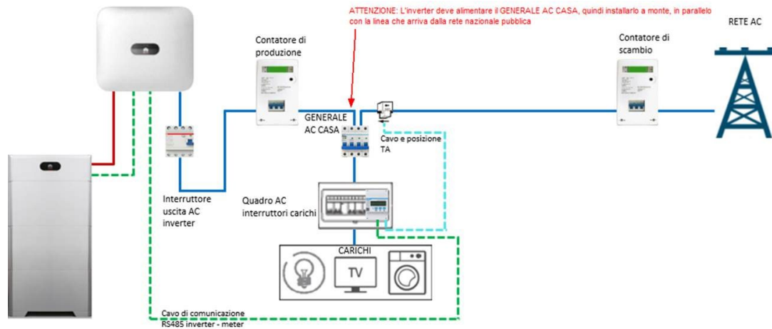
Figura 1.4: schema di posizionamento TA
