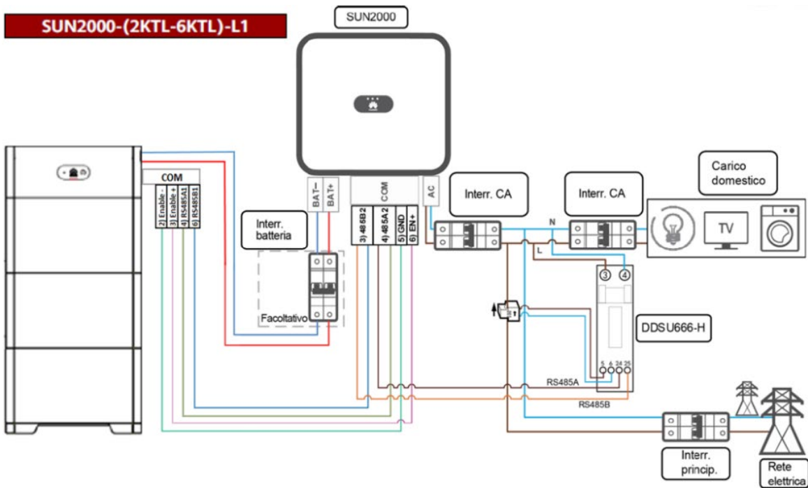
Figura 1.14: schema di connessione dei cavi COM per inverter monofase
